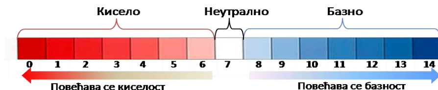
Слика 4.7. рН-скала
