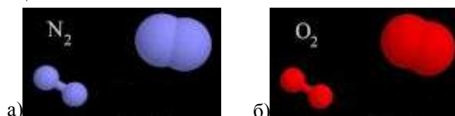
Слика 1.16. Модели и хемијске формуле молекула азота (а) и молекула кисеоника (б)
