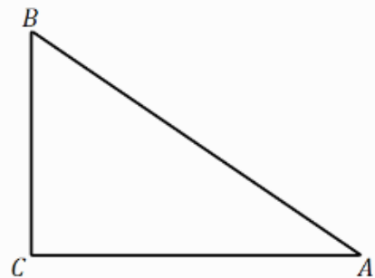
Slika 2. Pravougli trougao
