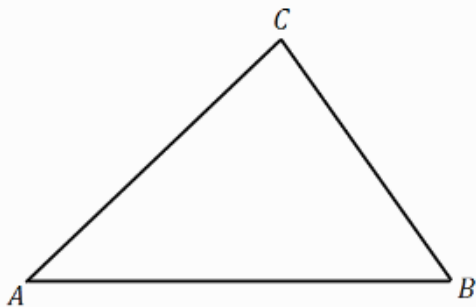
Slika 1. Oštrougli trougao
