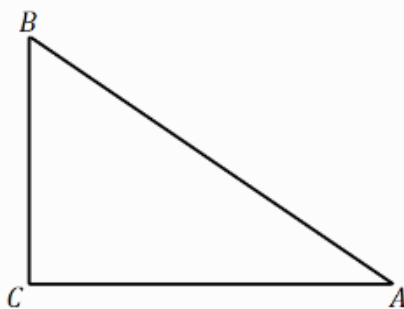
Slika 2. Pravougli trougao
